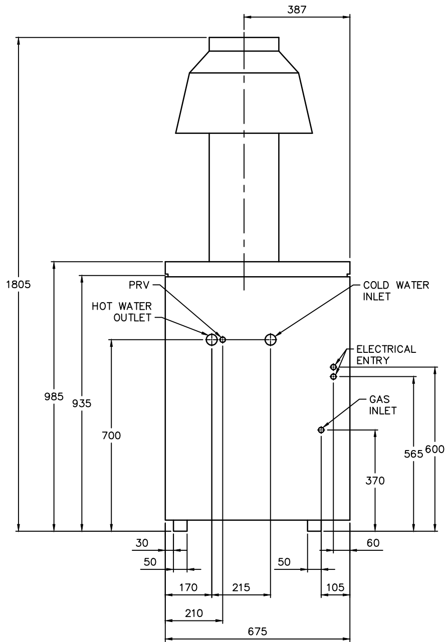
LEFT SIDE
