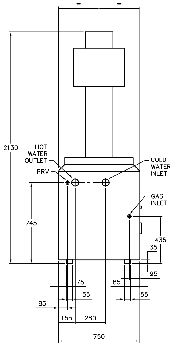
LEFT SIDE
